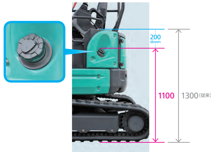
給油口位置 (単位:mm)
